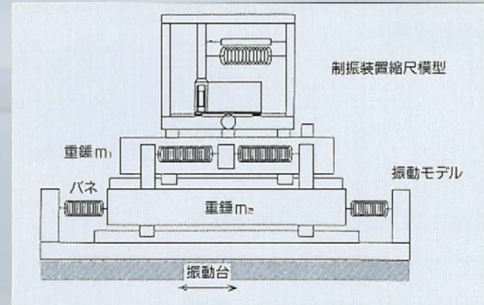
▶ 実験装置モデル図
